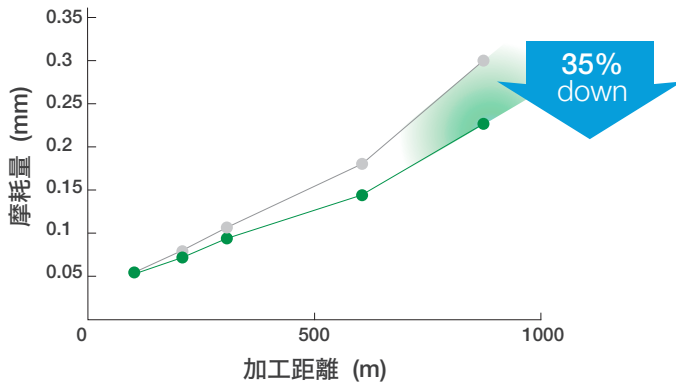
使用インサート：DCGT11 タイプ
