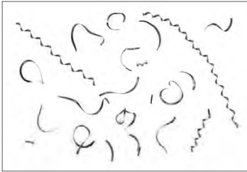
HF chipbreaker
